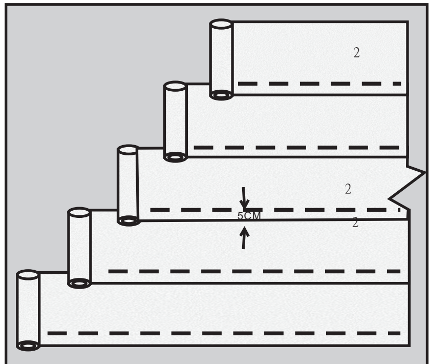
◎ 玻璃纖維網搭接示意圖 ◎
